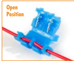
Insert wire
