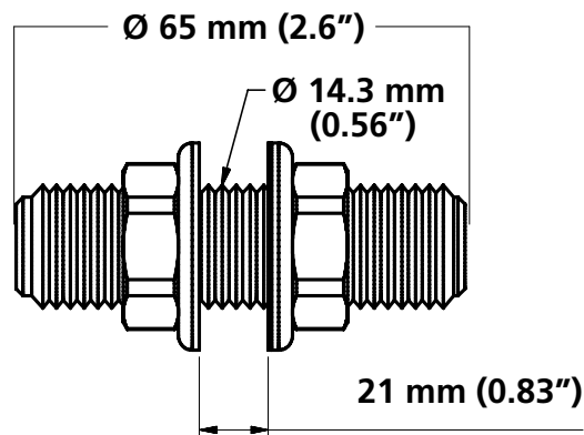
R7 DIMENSIONS
